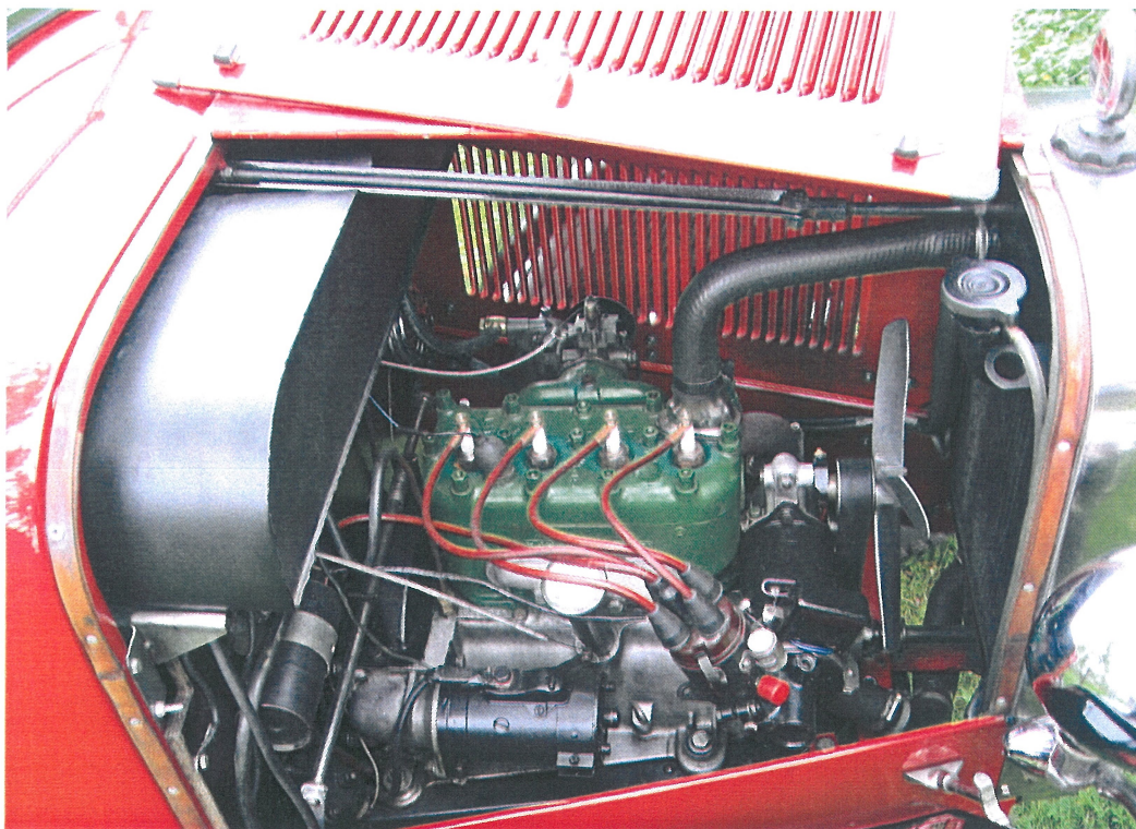
Vaade mootoriruumile vastassuunast
